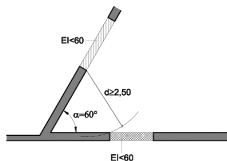
Figura 1.3. Fachadas a 60°
